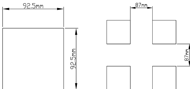
图 1 开孔尺寸及配电箱方孔间最小距离
