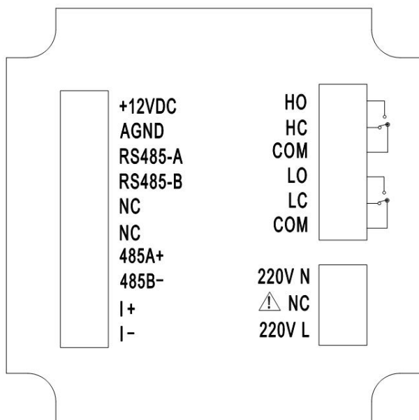
图 5 接线图
