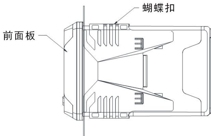
图 3 仪表安装示意图
