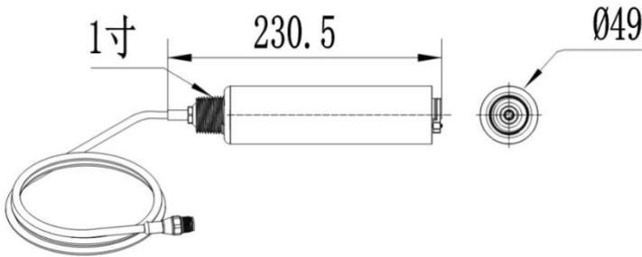
传感器外观尺寸
